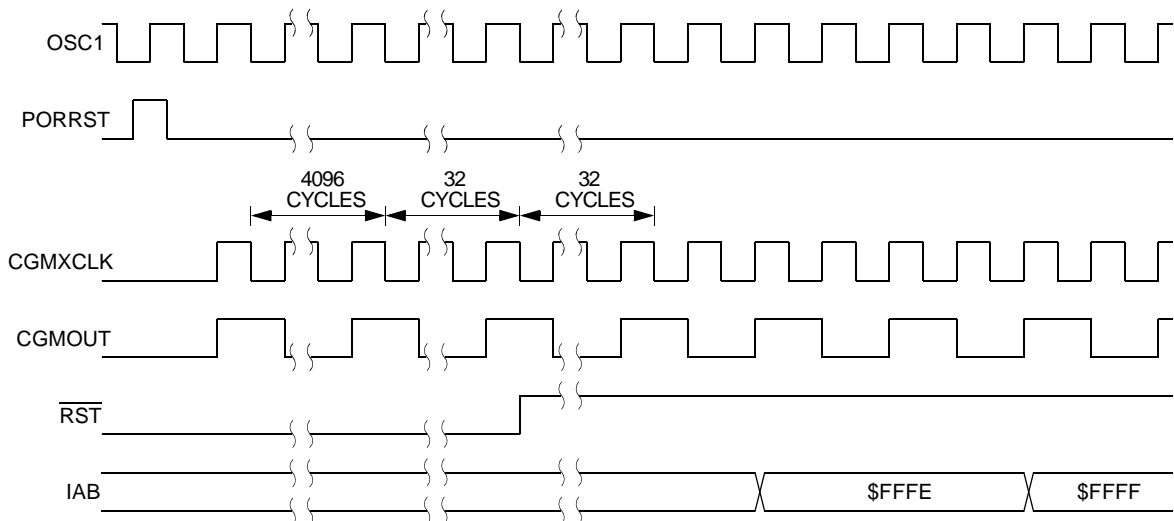
Figure 7-6. POR Recovery
