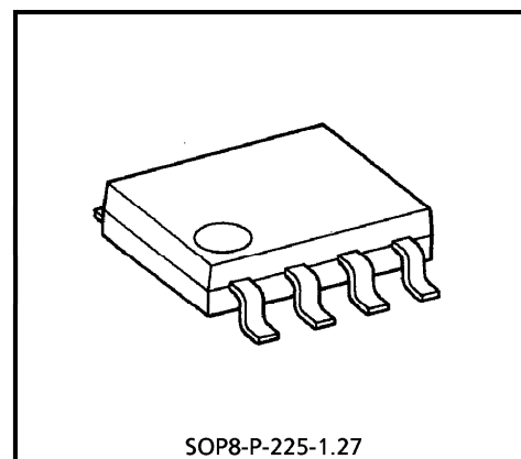
SOP8-P-225-1.27 Weight : 0.08g (Typ.)
