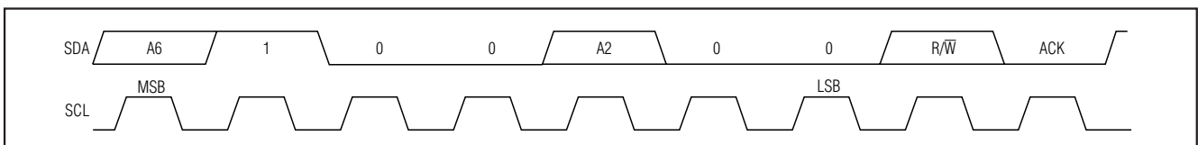
그림6. 슬레이브 주소
