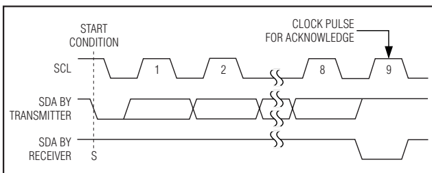
그림5. 승인
