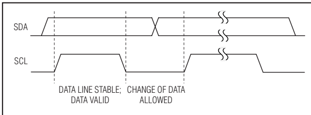
그림4. 비트 전송
