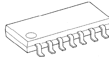
SOP14-P-225-1.27
