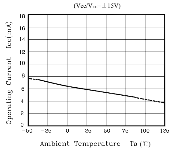
Fig. 8 I_{CC} - T_a
