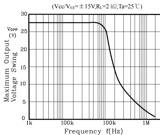
Fig. 2 V_{OP-P} - f
