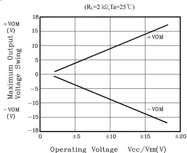
Fig. 4 V_{OM} - V_{CC}/V_{EE}
