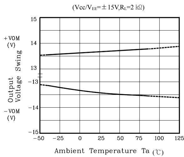
Fig. 7 V_{OM} - T_a
