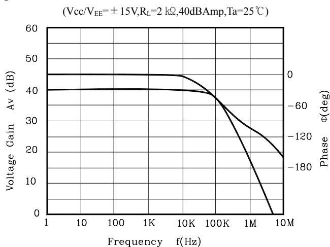
Fig. 1 G_V - f
