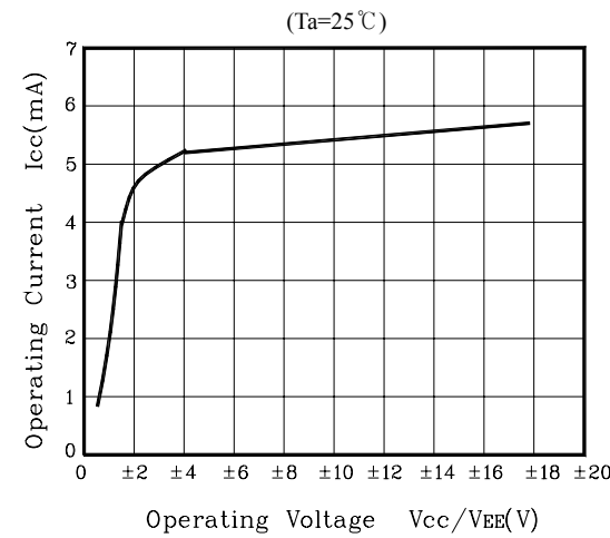
Fig. 10 I_{CC} - V_{CC}
