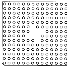
188 Pins 31
