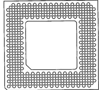
321 Pins A4
