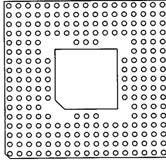
225 Pins 57
