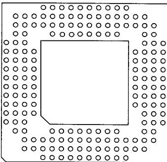
180 Pins 30
