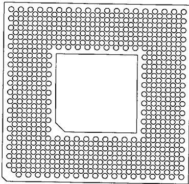
503 Pins A8
