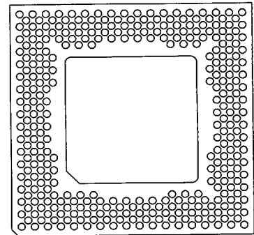
325 Pins A5 Without Window FP A2 TI TMS3200C40
