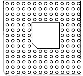
171 Pins 6
