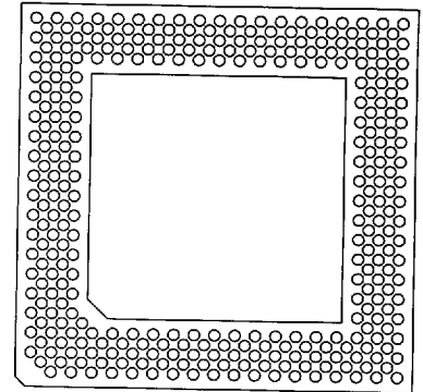
320 Pins A7 Without Window FP A5 Intel Pentium™ P54CM
