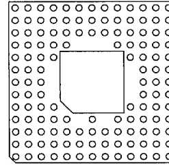
133 Pins 51
