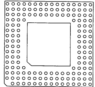
159 Pins 27
