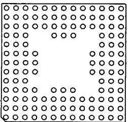
133 Pins 95
