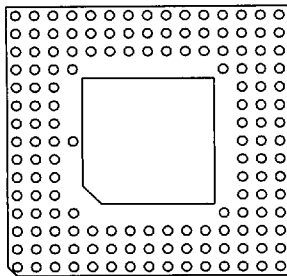
149 Pins 56
