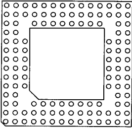
124 Pins 26
