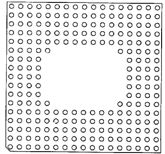
230 Pins 36
