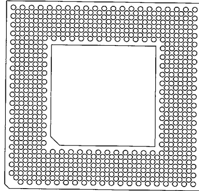
527 Pins A2
