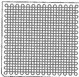
365 Pins A1
