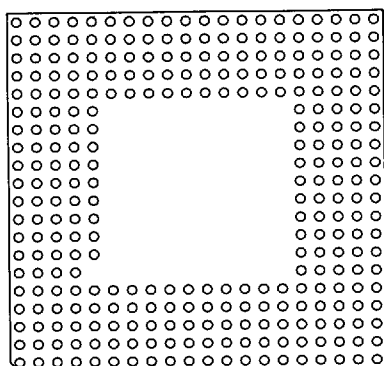
299 Pins 13
