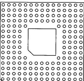
180 Pins 8
