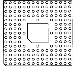
184 Pins 51
