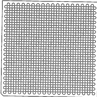
685 Pins A1
