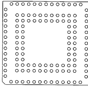
124 Pins 34
