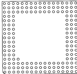
169 Pins 18
