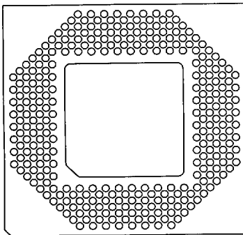
293 Pins A6
