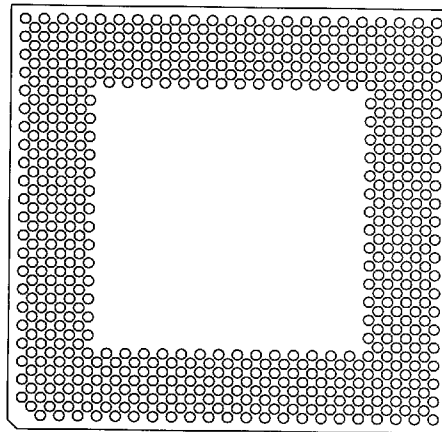
591 Pins A1
