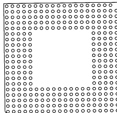
299 Pins 6
