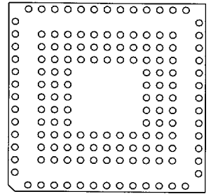
148 Pins 38
