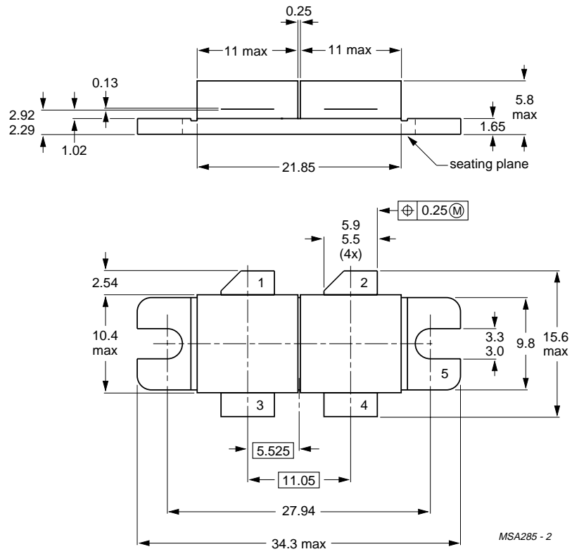
Fig.27 SOT262A1.
