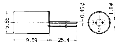
外形図-28
