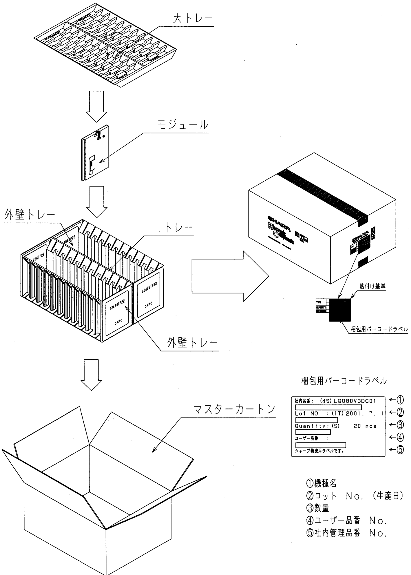
図3. 梱包形態図
