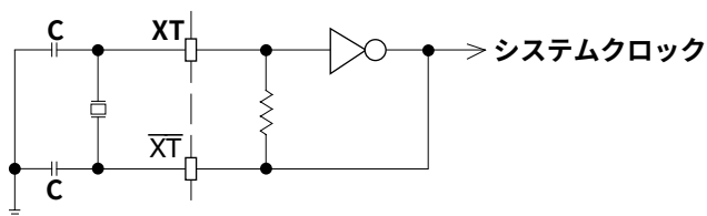
図-12 発振回路
