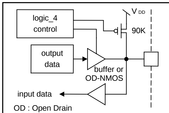
Input/Output IOC port : IOC3 - 0
