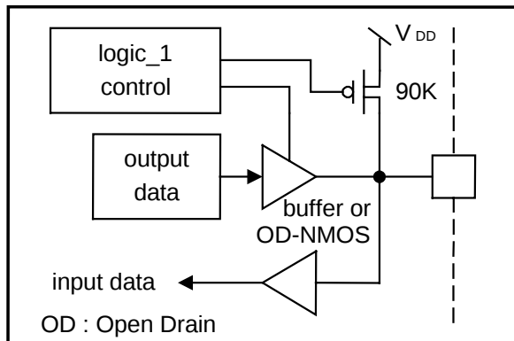
Input/Output IOA port : IOA3 - 0
