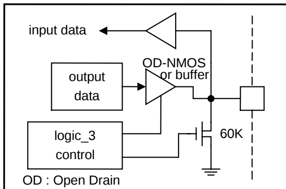
Input/Output IOB port : IOB5 - 4
