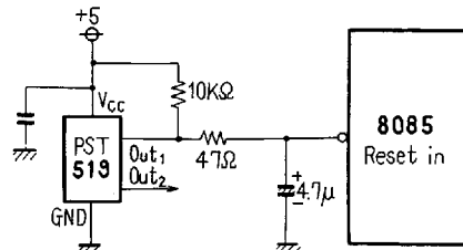
[Fig. 3] 8085 の Reset 回路/Reset circuit of 8085
