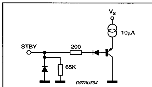
PIN: STBY
