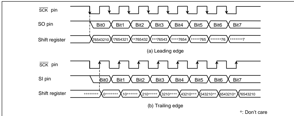
Figure 2.9.23 Shift Edge
