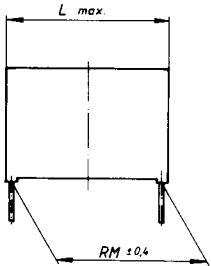
Ausf. / Fig. / ill. A
