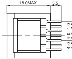
DIMENSIONS (mm) 外形寸法図
