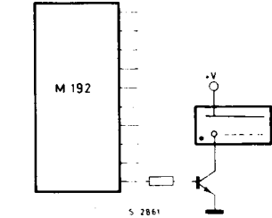
Fig. 5 - Gas discharge readout
