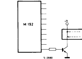
Fig. 4 - Incandescent readout
