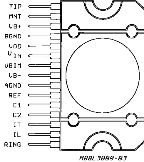
FLEXIWATT15
