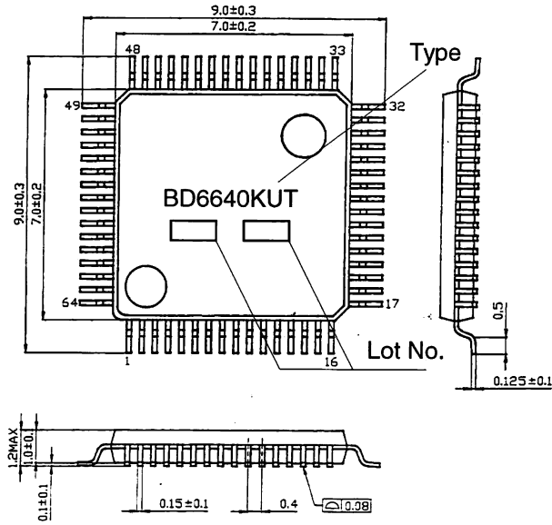
TQFP64U outlines (Unit : mm)
