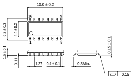
SOP16
