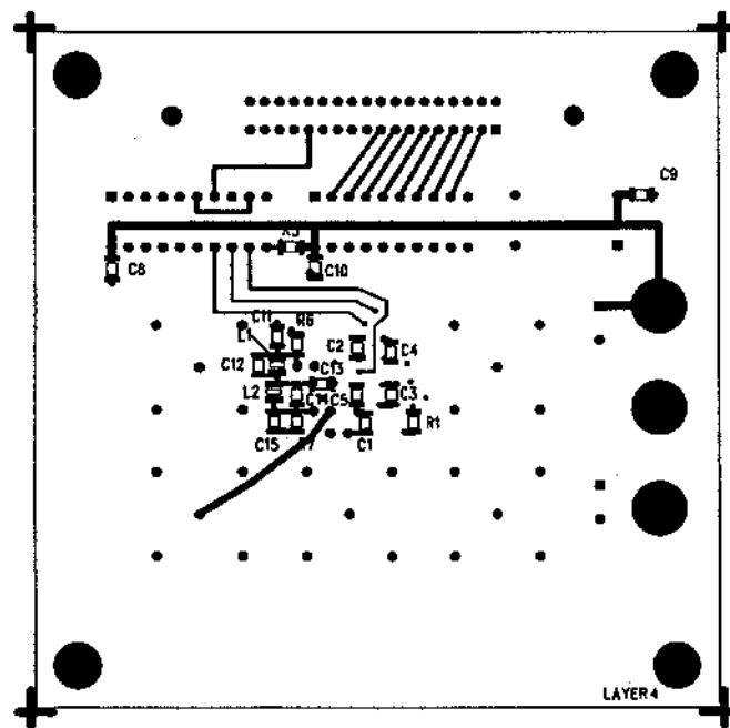
d. AD9850/CGPCB Bottom Layer
