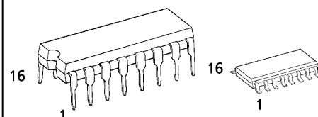
P (DIP16-P-300-2.54A) Weight : 1.00g (Typ.)
