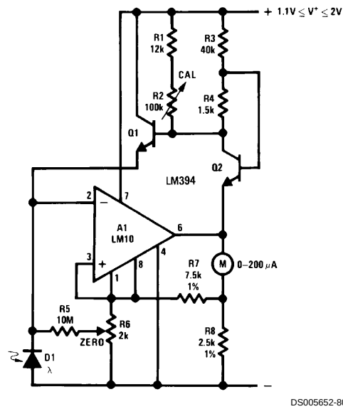
Light Meter
