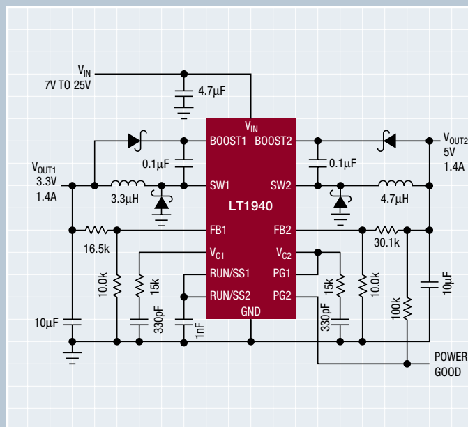
LT1940: Actual Size
