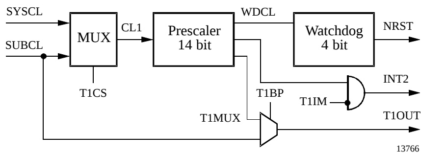
Figure 27. Timer 1 module
