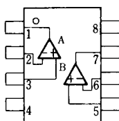
NJM2043D NJM2043M
