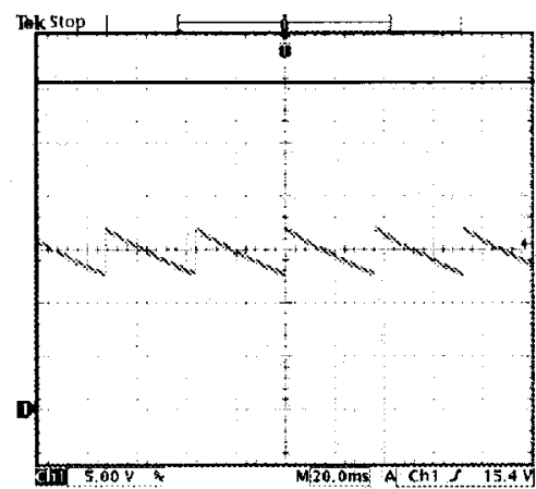
OVP Waveform
