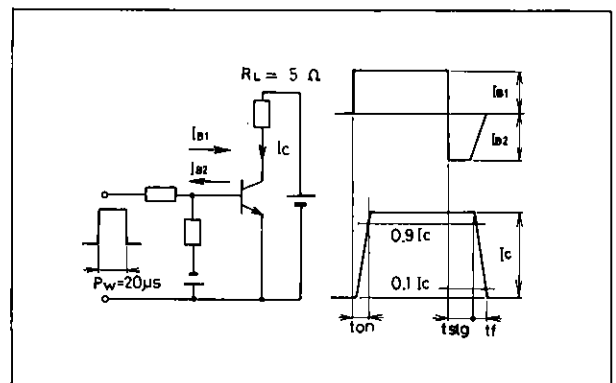
スイッチングタイム測定回路 *) Switching Time Test Circuit
