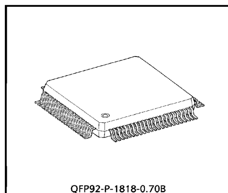
QFP92-P-1818-0.70B
