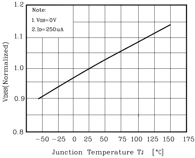
Fig. 7 V_{DSS} - T_J
