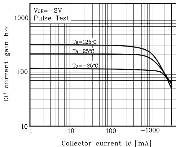
Fig. 4 h_{FE} - I_C
