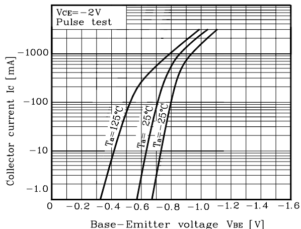
Fig. 2 I_C - V_{BE}
