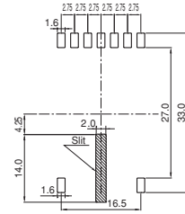
LAND PATTERNS (mm) 推奨ランド寸法
