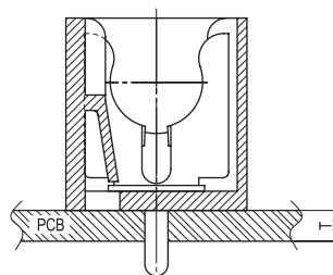
PCB ASS'Y
