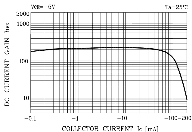
Fig. 1 h_{FE} - I_C
