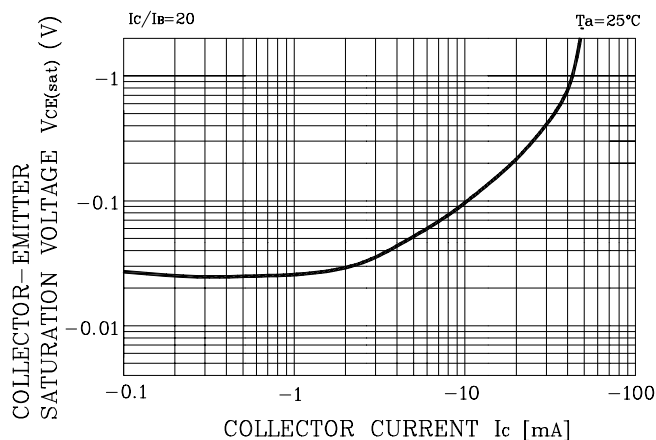
Fig. 2 V_{CE(SAT)} - I_C
