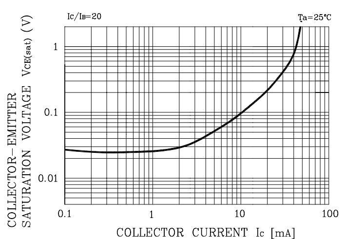
Fig. 2 V_{CE(SAT)} - I_C
