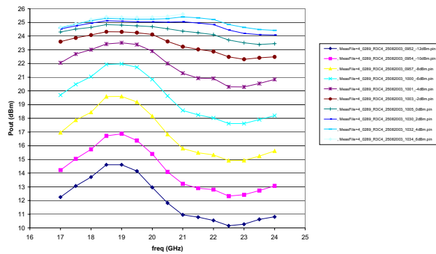
0289_R3C4 (Vd1 = 6.0V, Id1 = 50mA, Vd2 = 6.0V, Id2 = 90mA, Vd3 = 6.0V, Id3 = 180mA): Pout vs. freq
