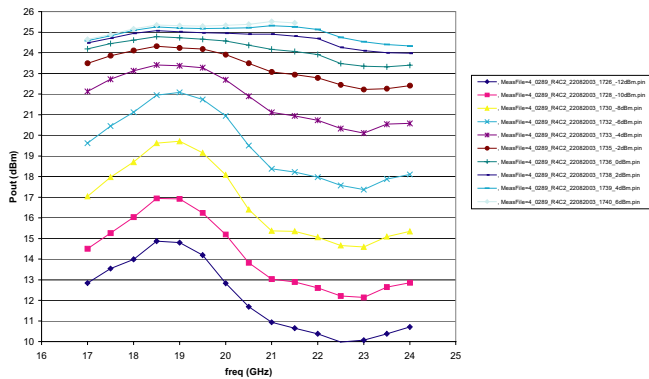
0289_R4C2 (Vd1 = 6.0V, Id1 = 50mA, Vd2 = 6.0V, Id2 = 90mA, Vd3 = 6.0V, Id3 = 180mA): Pout vs. freq
