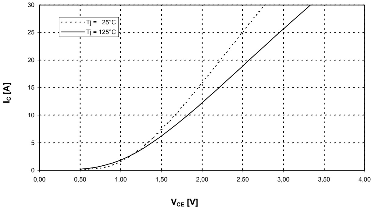
Ausgangskennlinienfeld Brems-Chopper-IGBT (typisch) I_C = f(V_{CE}) output characteristic brake-chopper-IGBT (typical) V_{GE} = 15\text{ V}
