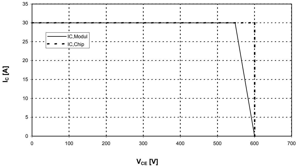
Sicherer Arbeitsbereich Wechselr. (RBSOA) I_C = f(V_{CE}) reverse bias safe operating area inverter (RBSOA) T_{vj} = 125^\circ\text{C} , V_{GE} = \pm 15\text{V} , R_G = 68 \text{ Ohm}
