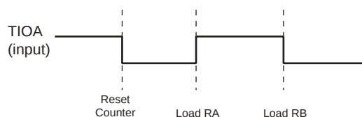
Figure 94. TIOA Pulse or Period
