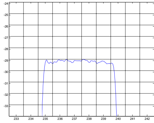
Phase Linearity( f_0 \pm 2.4 MHz)
