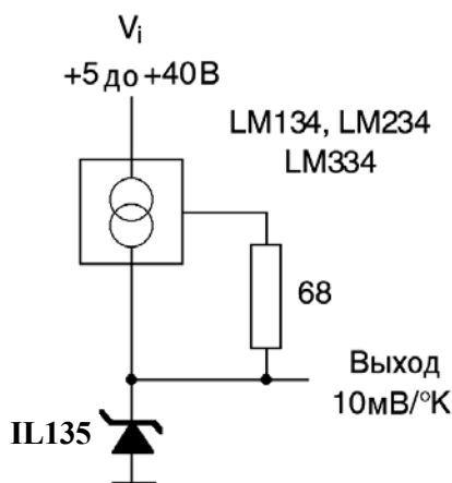
Рисунок 15 – Схема применения с широким диапазоном напряжения питания
