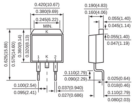
D2PAK
