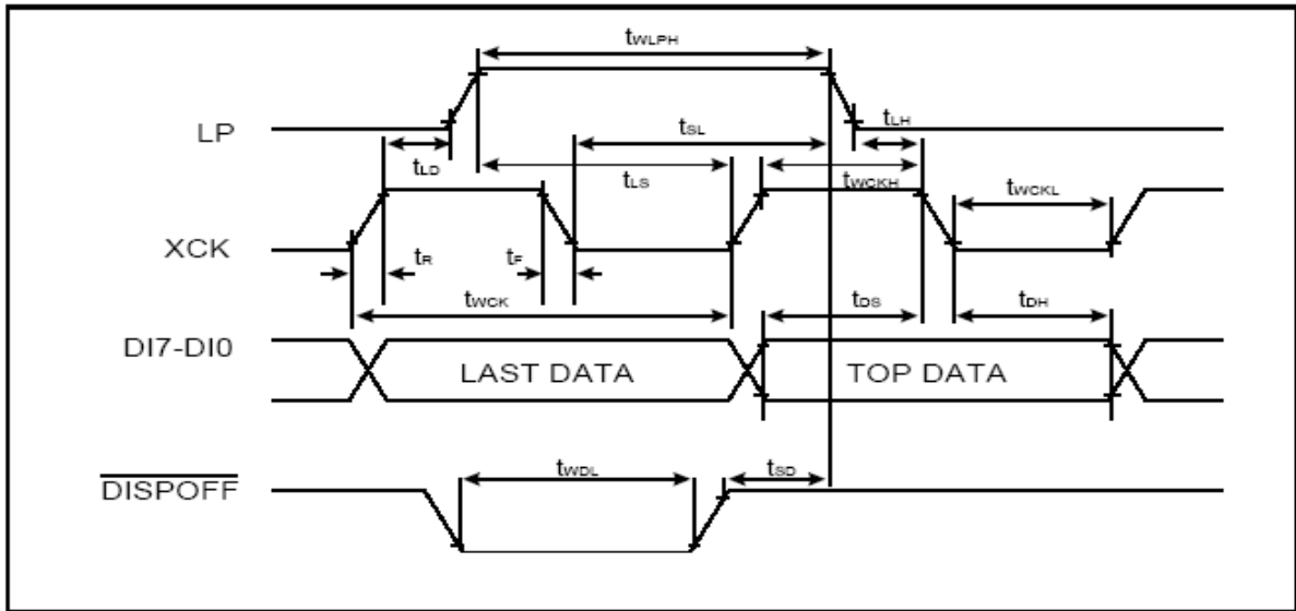
图 A-1: Segment 模式的时序特性波形图
