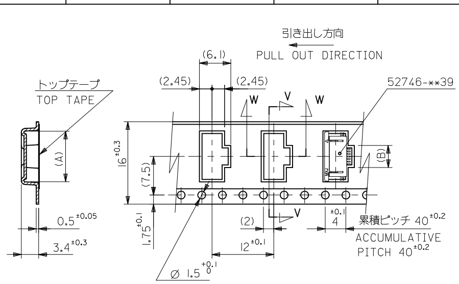
SECT.V-V
