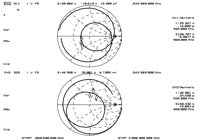
Zin, Zout
