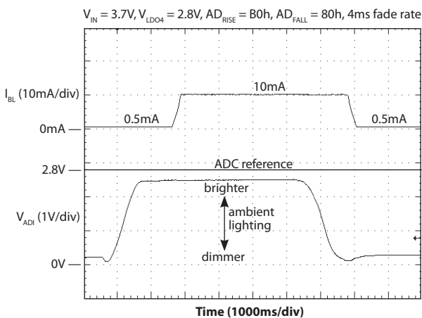
Backlight Dimming with ALS and Fade
