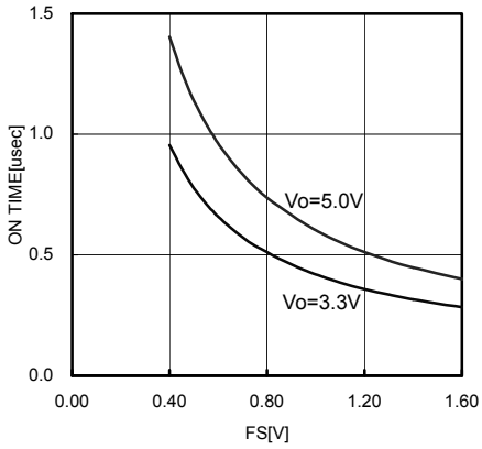
Fig. 13 FS-ON TIME
