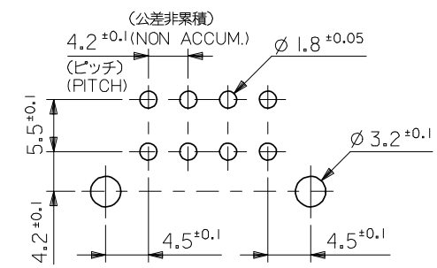
基板穴推奨寸法 RECOMMENDED P.C. BOARD PATTERN
