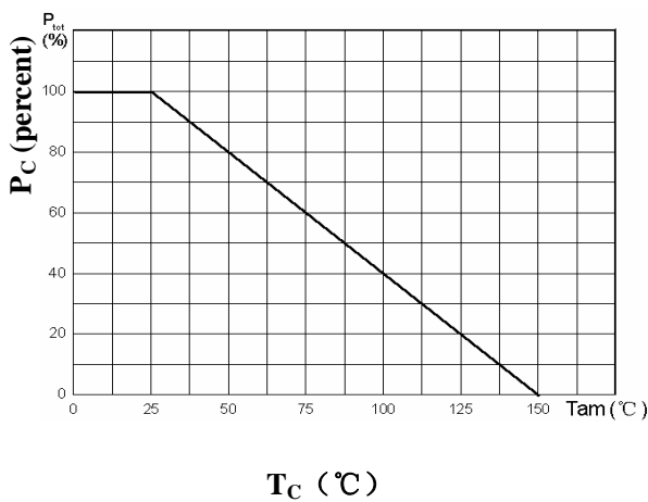
P_C - T_C
