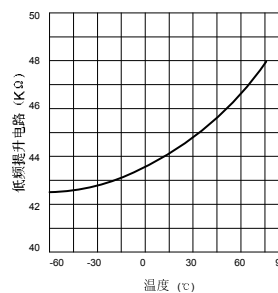
图15 低音提升电阻和温度关系特性曲线
