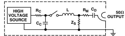
Figure 12. EFT Generator
